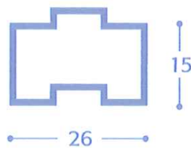
ART. 48 PROFILO DI COMPENSAZIONE
