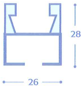
ART. 44 GUIDA DI SCORRIMENTO E ATTACCHI LATERALI
