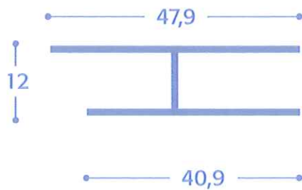
ART. 49 PROFILO PER BATTUTA PER APERTURA CENTRALE
