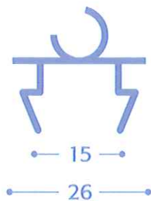
ART. 45 PROFILATO A SCATTO PARTENZA
