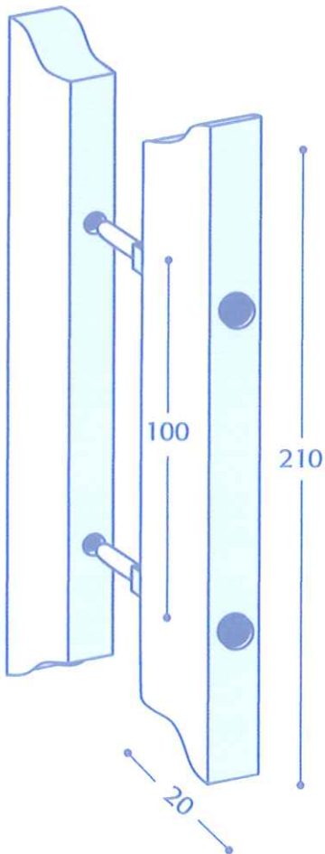
MANIGLIA IN PVC CON CALAMITA
